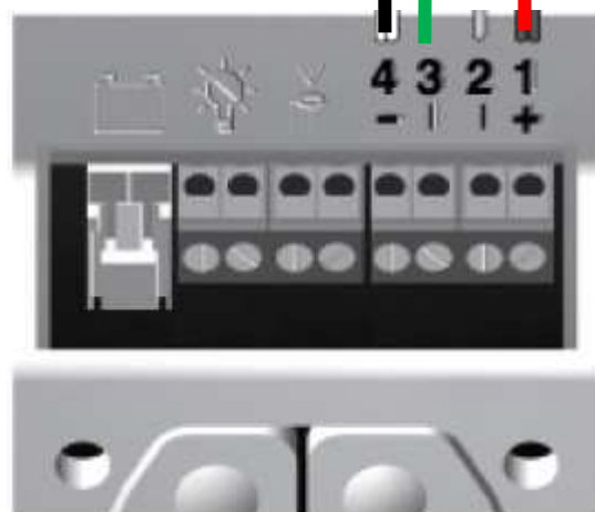
Bornier Moteur
