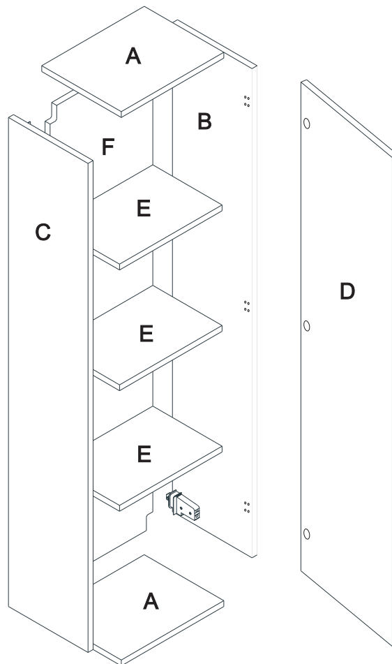
H8 3xM4x22
