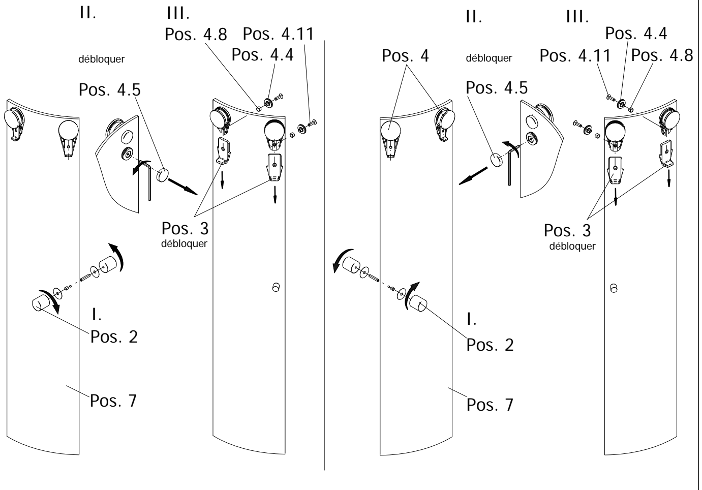
montage de la porte sans joint bas
