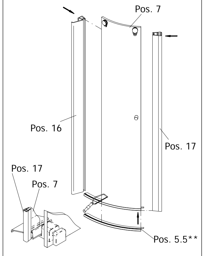
montage de la porte avec joint bas
