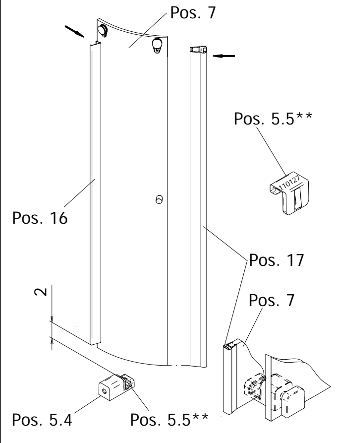
montage de la porte sans joint bas
